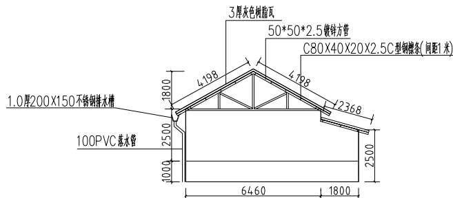
1-1剖面图
