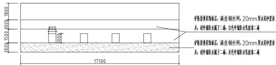
A立面
