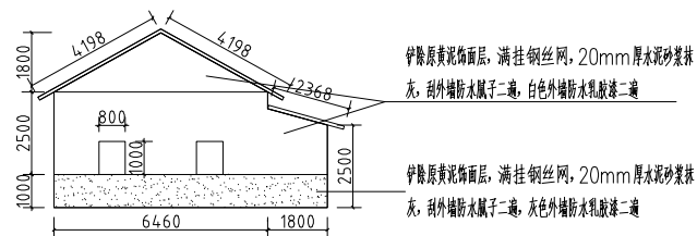
D立面
