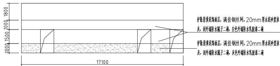
C立面
