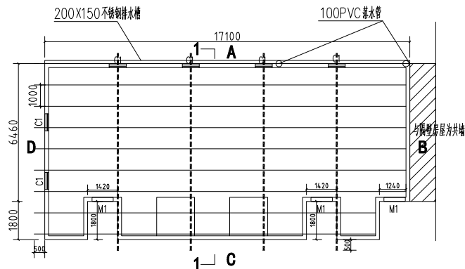
屋面平面图
